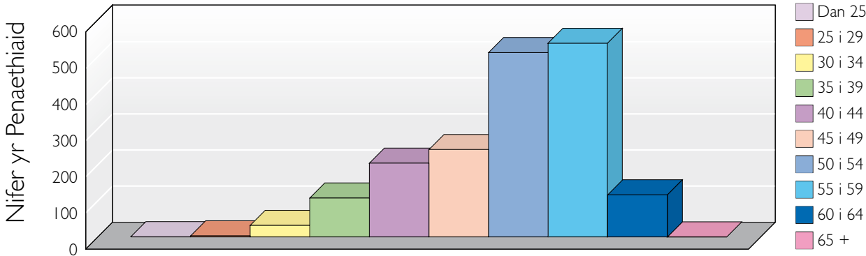
Mawrth 2007
