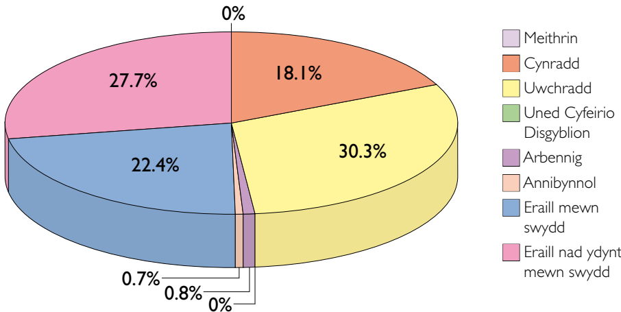
Mawrth 2007
