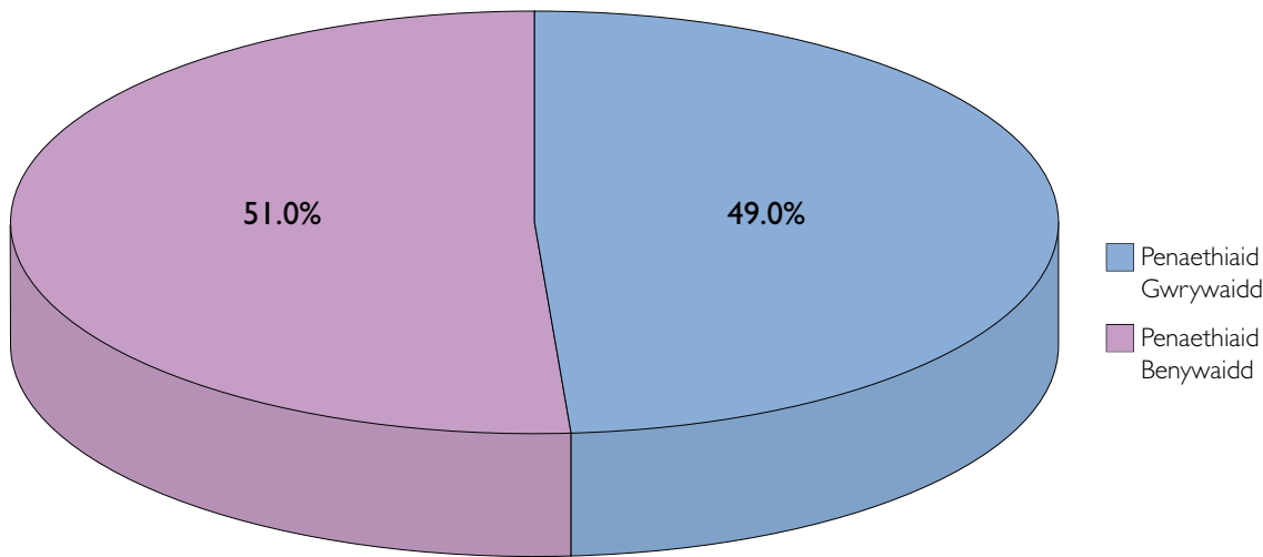
Mawrth 2007
